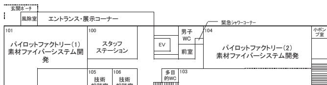
ファイバーイノベーション・インキュベーター施設1階平面図
